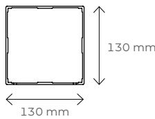
Przekrój słupa
