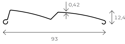
Przekrój lameli Z90 [mm]
