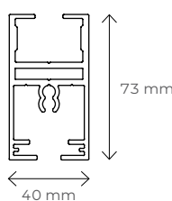
Przekrój ramy górnej
