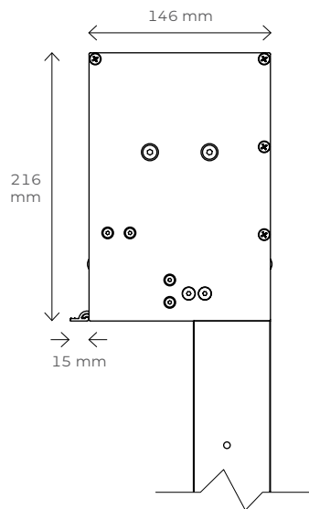
Wymiar kasety BOX 1
