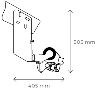
Montaż do krokwi dachowej
