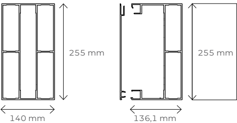
Przekrój belki skrajnej i pośredniej
