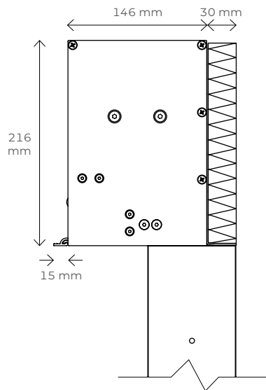
Wymiar kasety BOX 2
