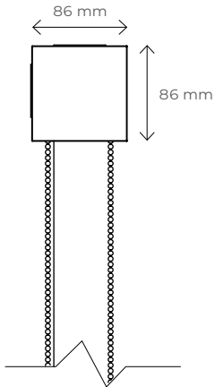
Wymiar kasety 85 SA / MA
