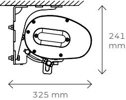
Montaż do sufitu
