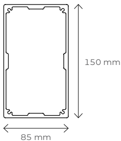
Przekrój słupa
