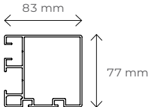
Przekrój prowadnicy
