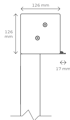
Wymiar kasety 120 Ziip DZ (do zabudowy)
