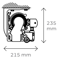
Montaż do sufitu
