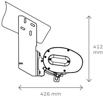
Montaż do krokwi dachowej
