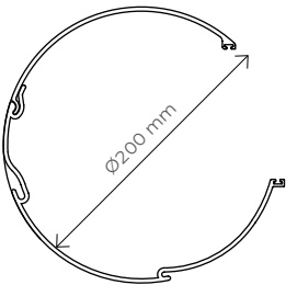
Przekrój kasety
