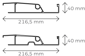
Przekrój pióra STANDARD (typ FLAT)
