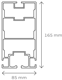
Przekrój prowadnicy
