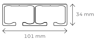
Przekrój prowadnicy dwutorowej górnej
