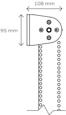
Wymiary uchwytu ścienno-sufitowego XL MA
