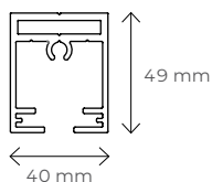
Przekrój ramy bocznej i dolnej
