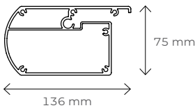
Przekrój prowadnicy
