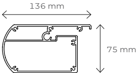
Przekrój belki przedniej
