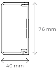
Przekrój prowadnicy
