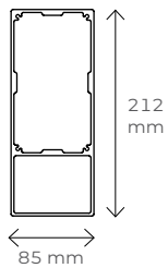
Przekrój belki z widocznym silnikiem
