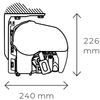
Montaż do sufitu
