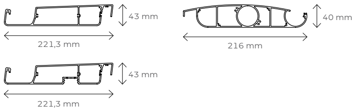
Przekrój piór
