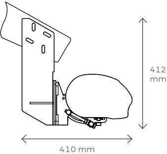
Montaż do krokwi dachowej
