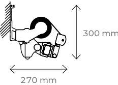
Montaż do ściany
