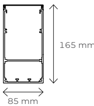
Przekrój belki
