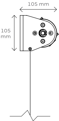
Wymiary uchwytu ścienno-sufitowego XL
