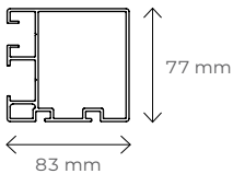
Przekrój prowadnicy
