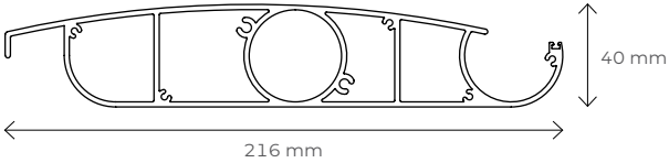
Przekrój pióra
