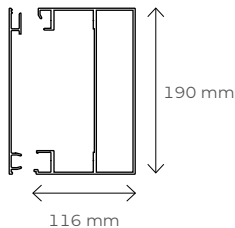
Przekrój belki
