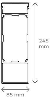
Przekrój belki z ukrytym silnikiem
