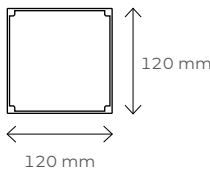
Przekrój słupa
