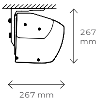
Montaż do sufitu
