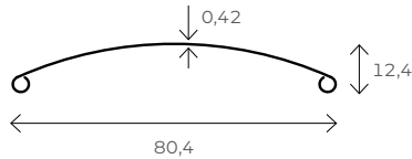
Przekrój lameli C80 [mm]
