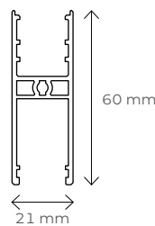
Przekrój ramy dolnej
