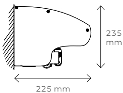
Montaż do ściany opcja z daszkiem
