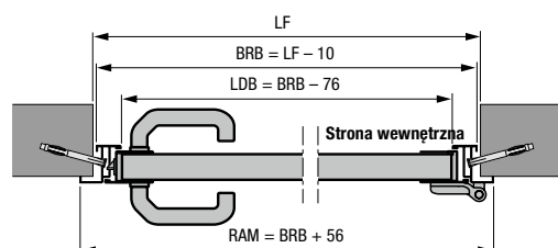
Drzwi boczne z aluminiową ościeżnicą kątową, profil typu 2 Mocowane od wewnątrz
