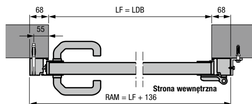
Drzwi boczne z aluminiową ościeżnicą blokową, profil typu 2 Montaż za otworem
