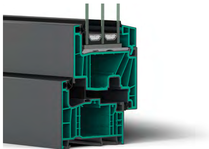
Materiały z recyklingu w rdzeniu profilu ARTEVO i listwach przyszybowych
